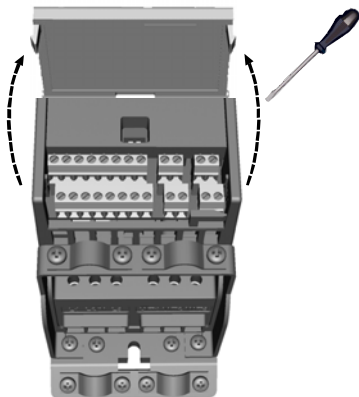
Рис. 14. Откройте крышку MI1–MI3
