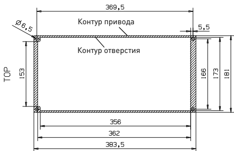
Рис. 5. Размеры выреза для фланцевого крепления приводов типоразмеров MI4 (ед. изм.: мм)
