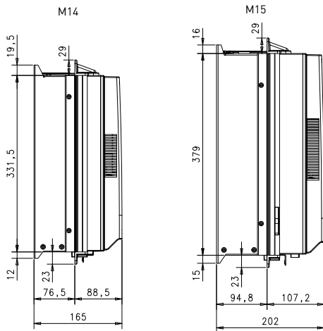
Рис. 7. Размеры углубления для фланцевого крепления приводов типоразмеров M14 и M15 (ед. изм.: мм)
